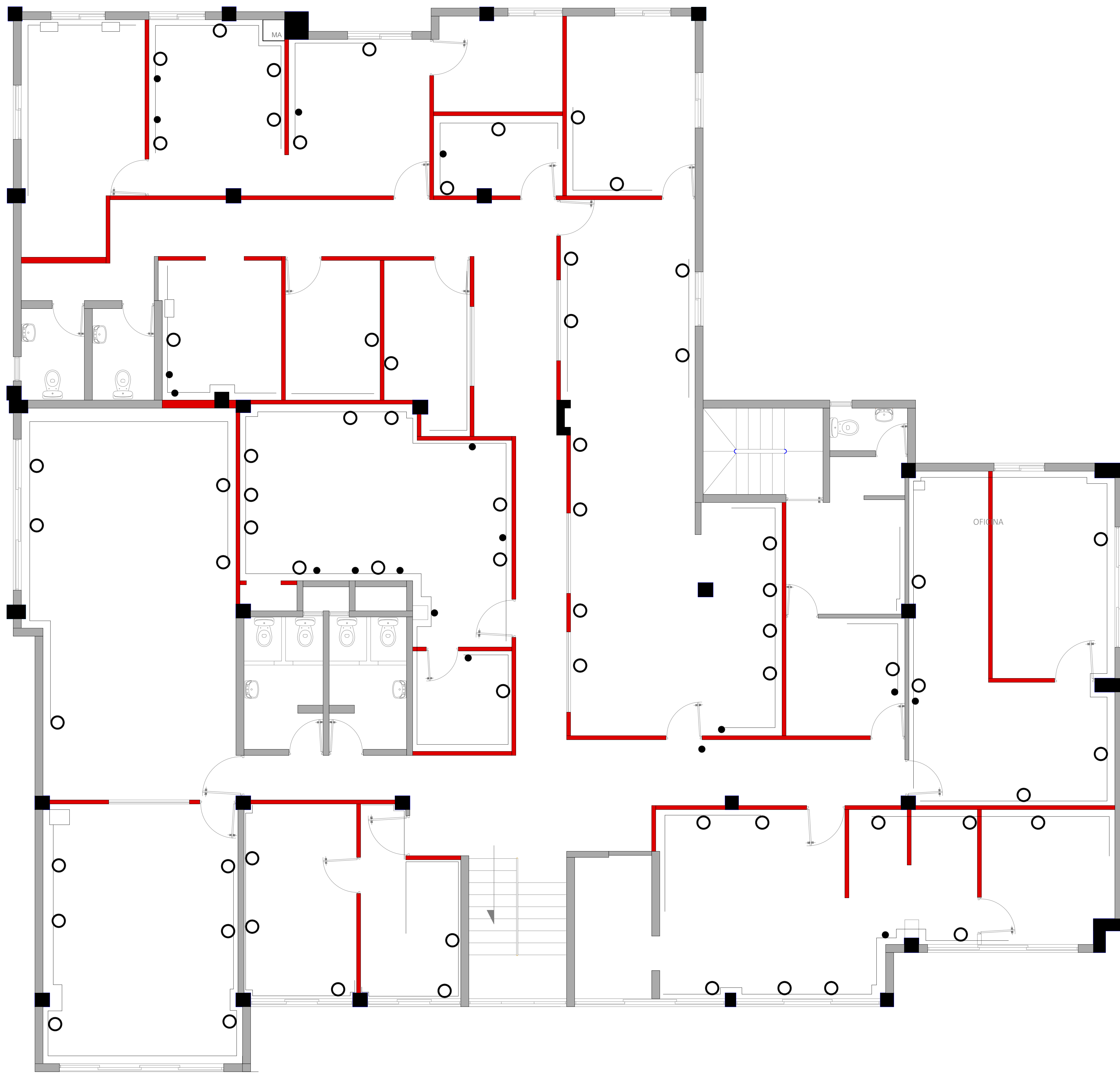
PLANTA DE TRABAJO - DEMOLICIÓN TERCER NIVEL ESC.:1:50
