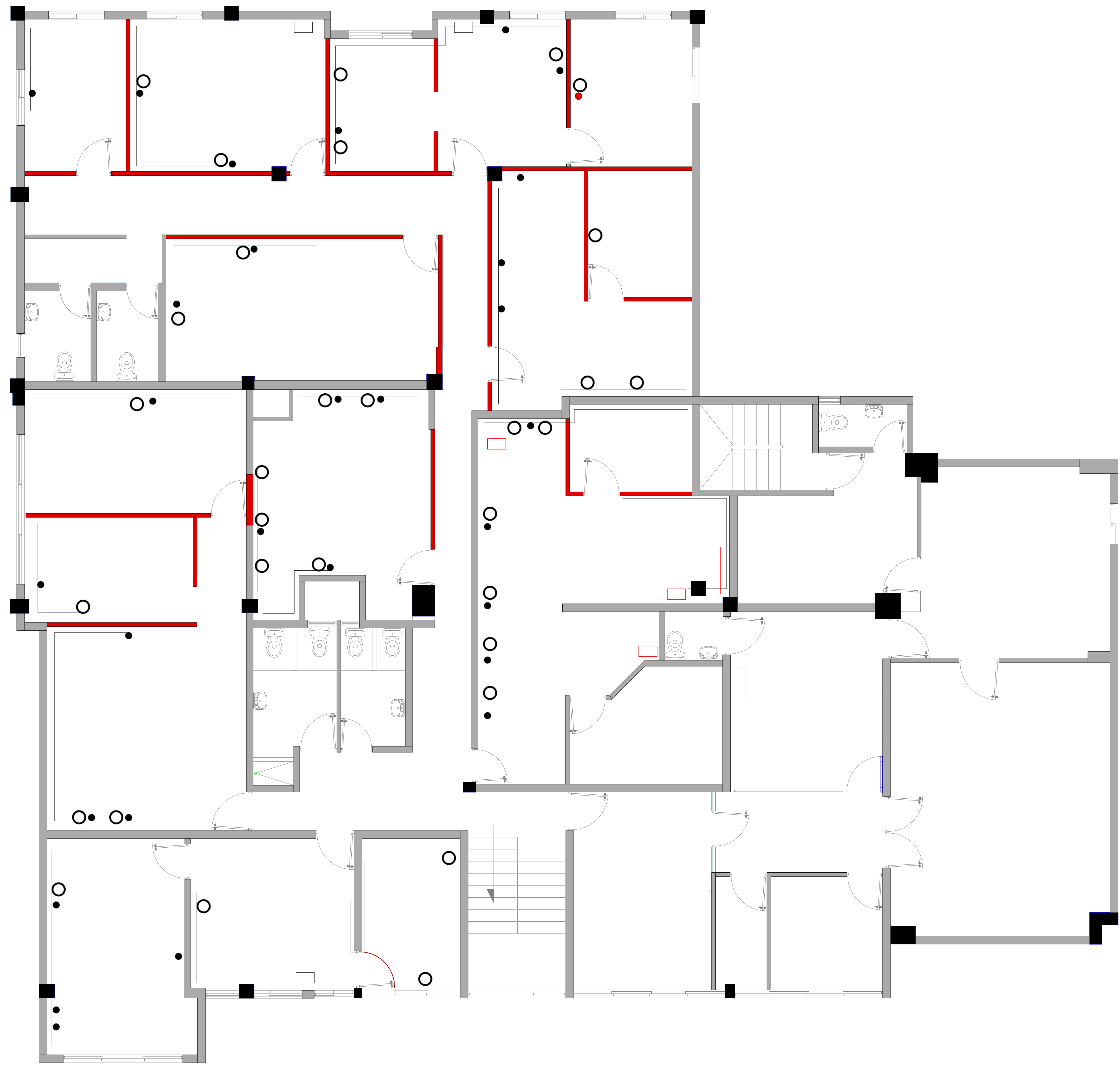
PLANTA DE TRABAJO - DEMOLICIÓN SEGUNDO NIVEL ESC.:1:50
