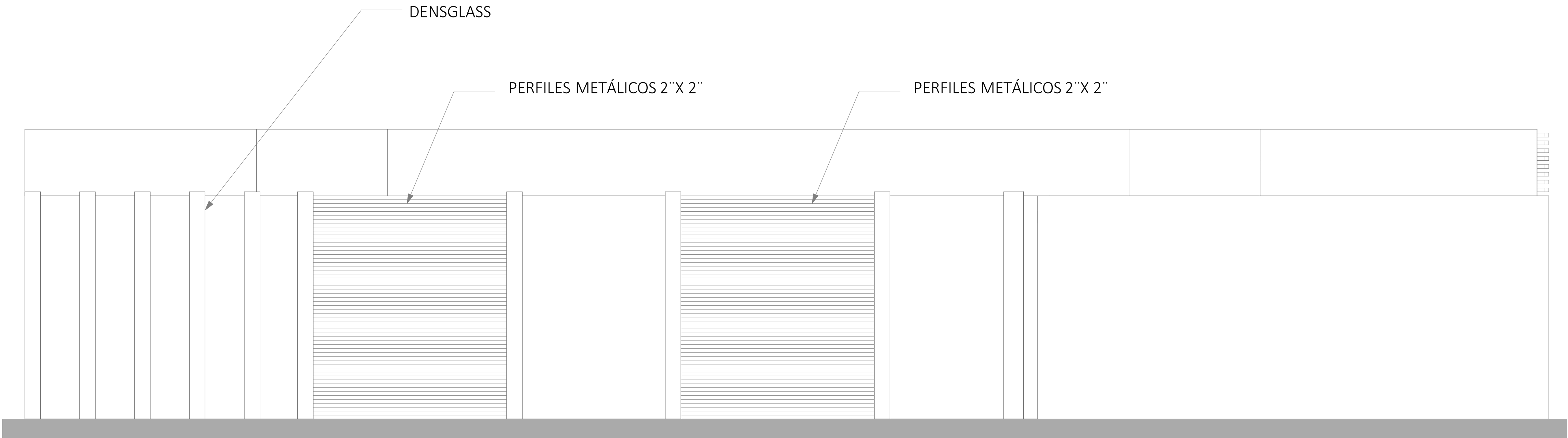
A-18-1 ELEVACIÓN POSTERIOR DISPENSARIO INSTITUTO NACIONAL DE TRÁNSITO Y TRANSPORTE TERRESTRE - INTRANT SCALE: 1:33
