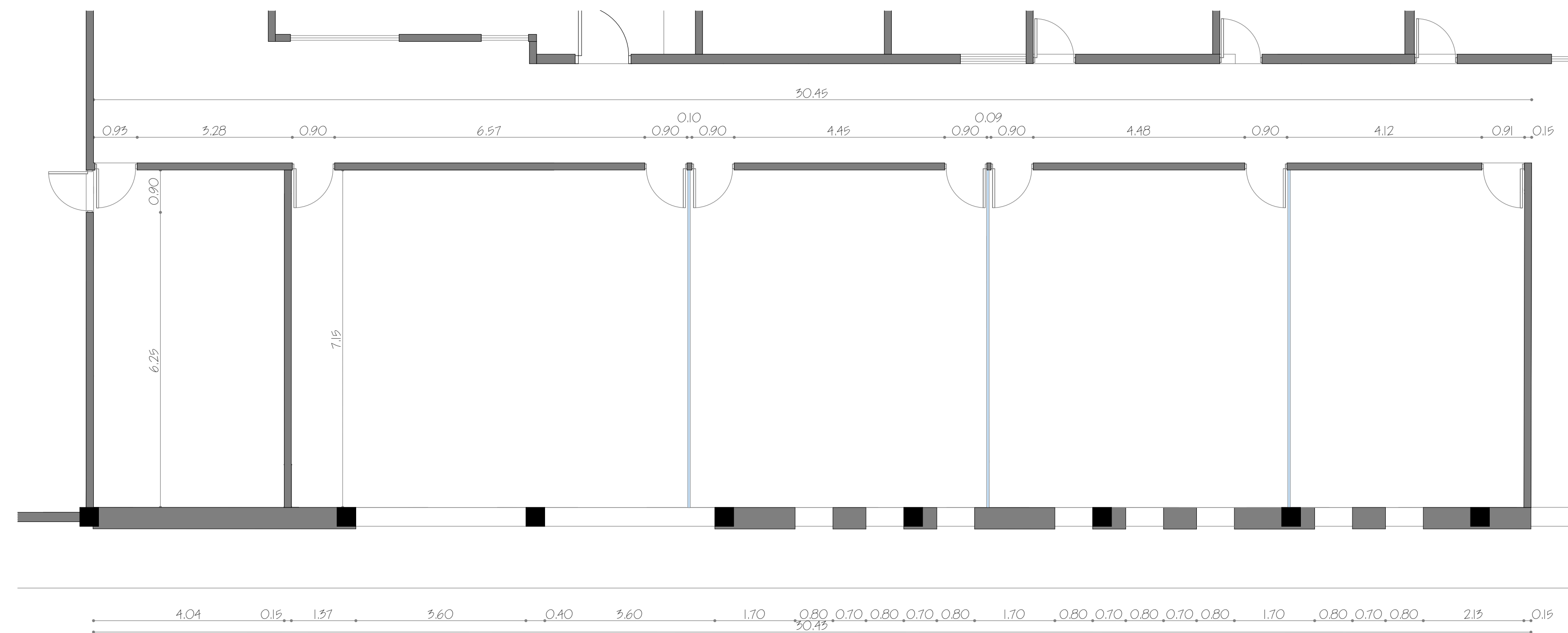
A-18-2 ACERCAMIENTO HANGAR INSTITUTO NACIONAL DE TRÁNSITO Y TRANSPORTE TERRESTRE - INTRANT SCALE: 1:75
